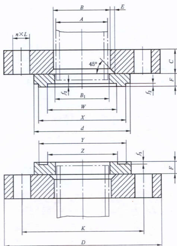
图3 榫槽面(TG)平焊环板式松套钢制管法兰 (适用于 PN 10、PN 16、PN 25 和 PN 40)
